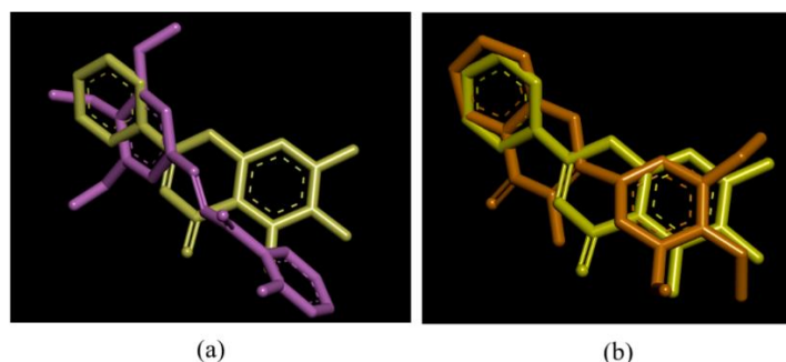
Gambar 10. Visualisasi overlay pose pengikatan ligan menggunakan perangkat lunak DSV 2021, (a) senyawa C 345 (ungu) dengan baicalein (kuning), (b) senyawa F 345 (jingga) dengan baicalein (kuning).
